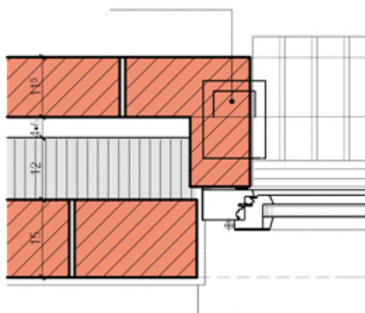
Grundriss Leibung
